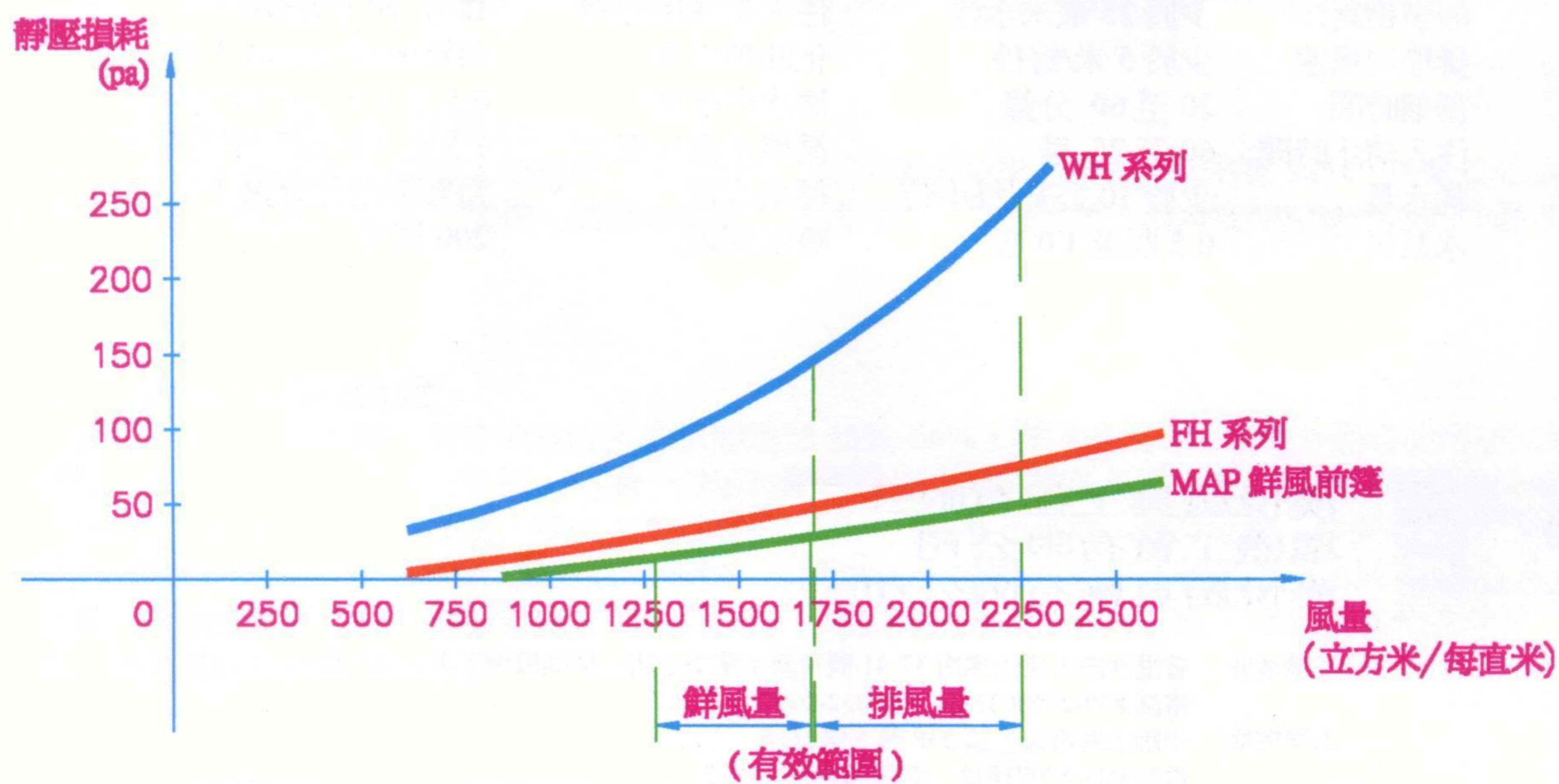
靜壓損耗 / 風量關係曲線
