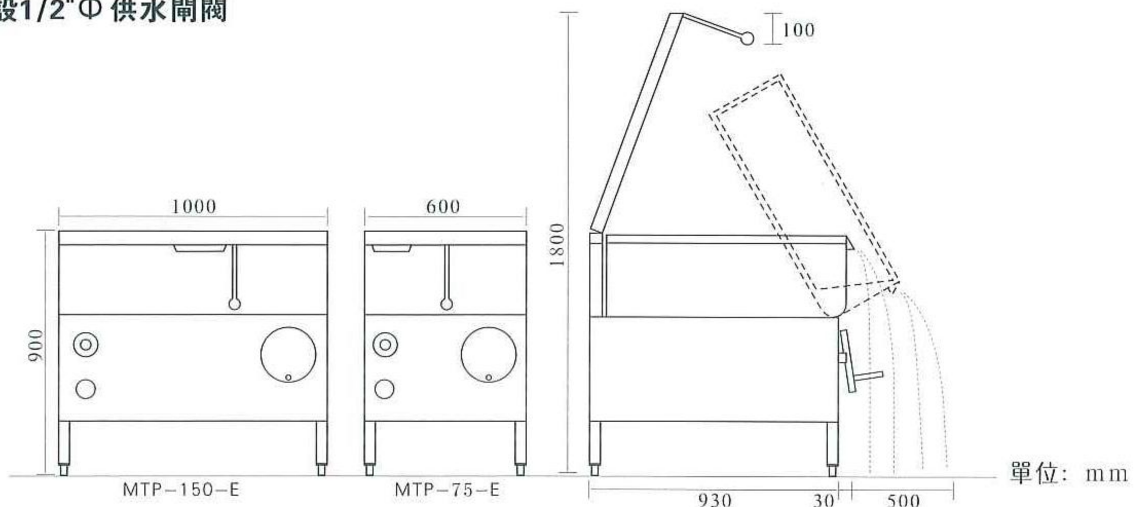
型號(Model):MTP-150-E
